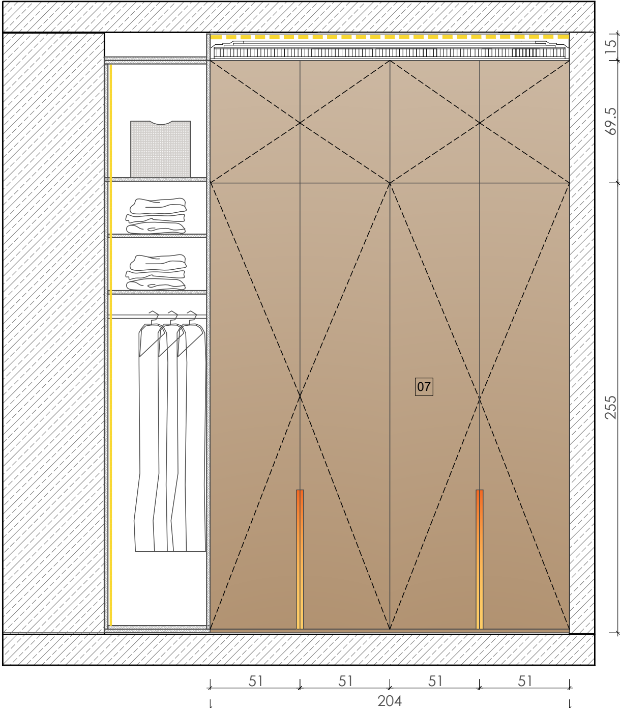
PRZEKRÓJ D-D
