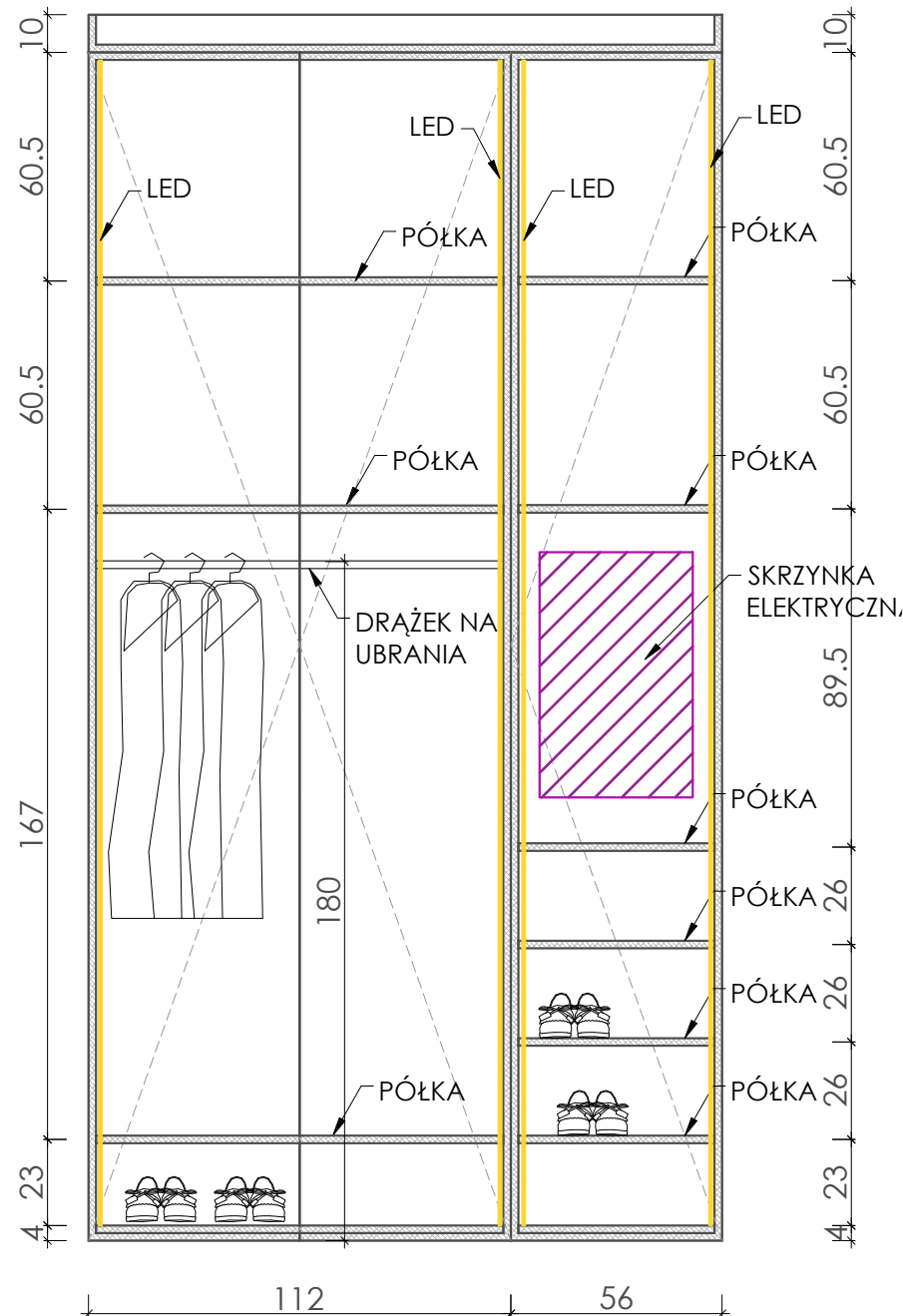
WNĘTRZE SZAFY
