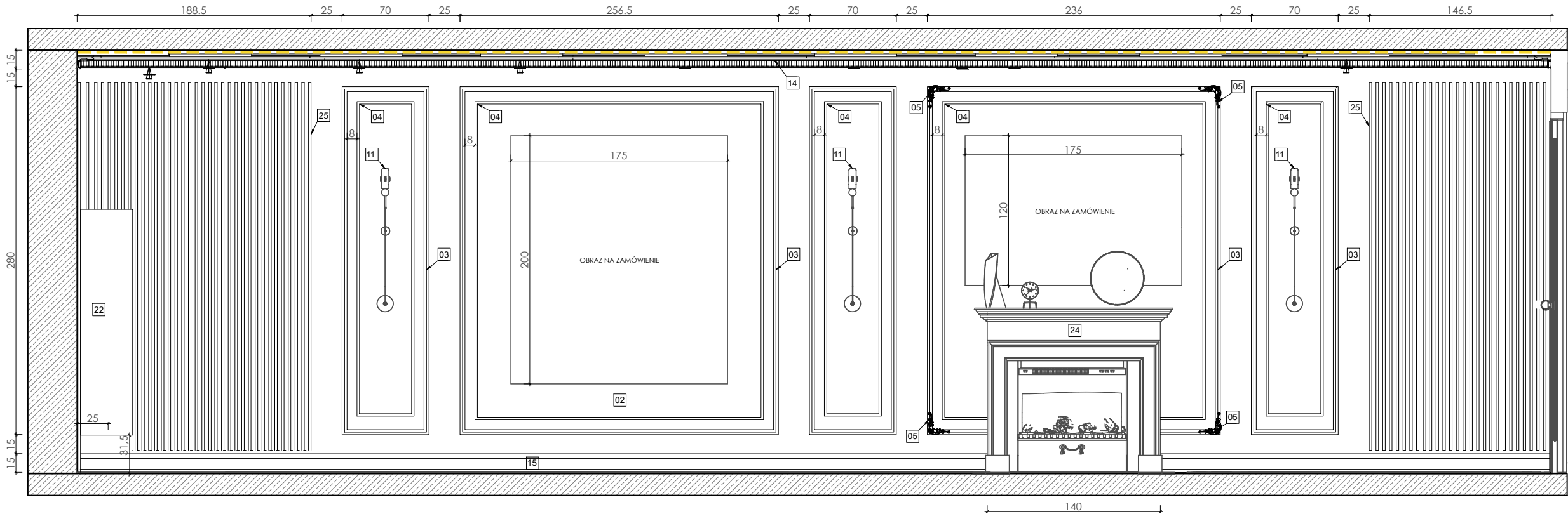
PRZĘKRÓJ B-B
