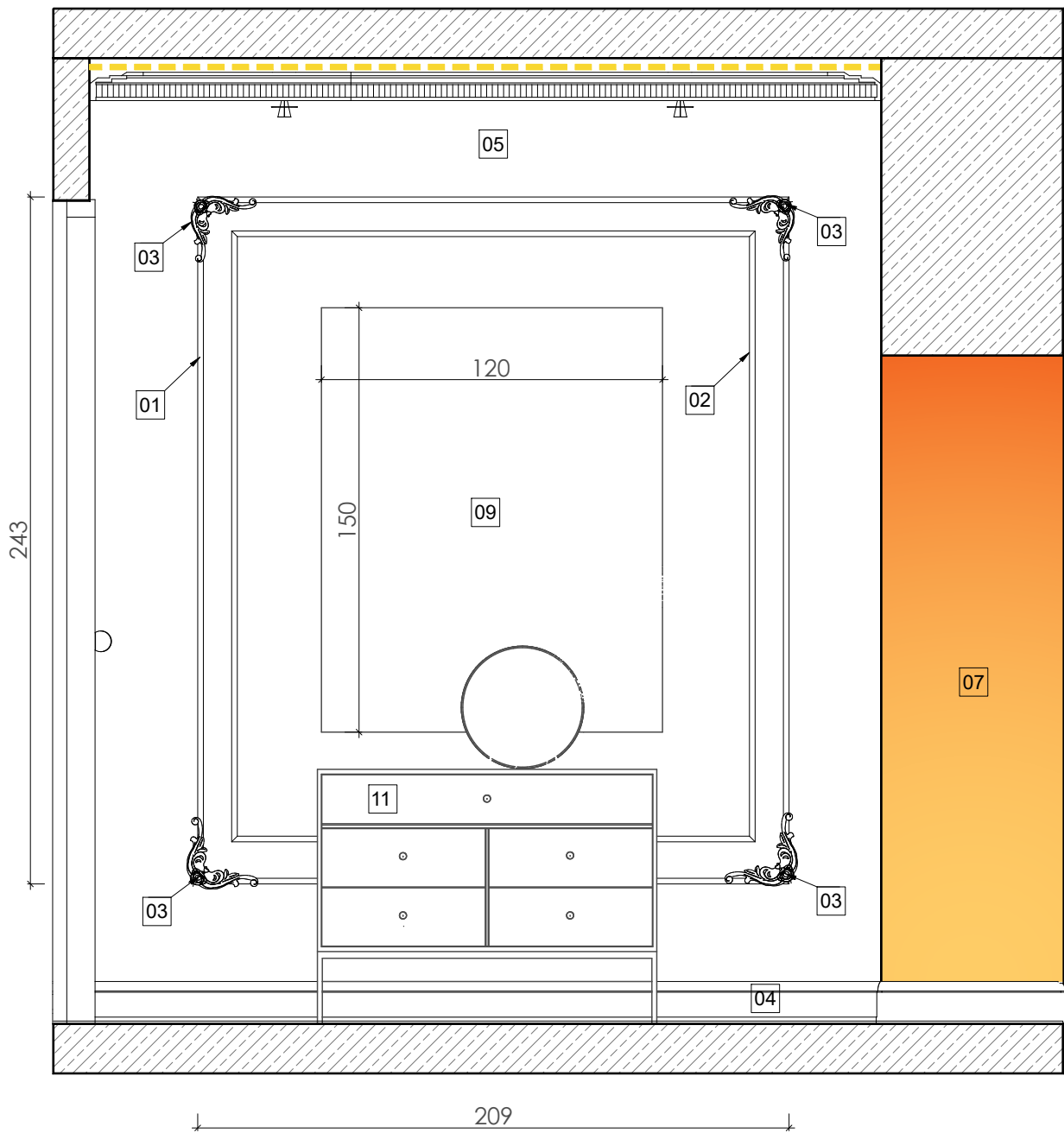
PRZEKRÓJ B-B
