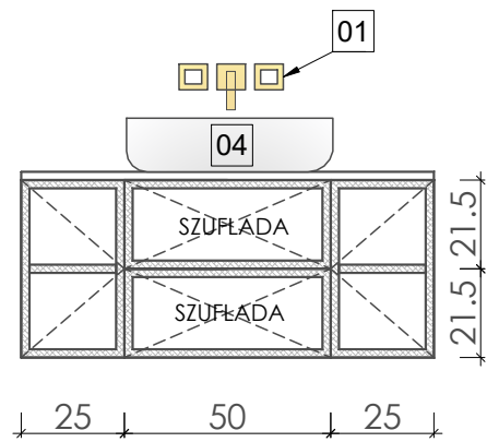
RZUT
