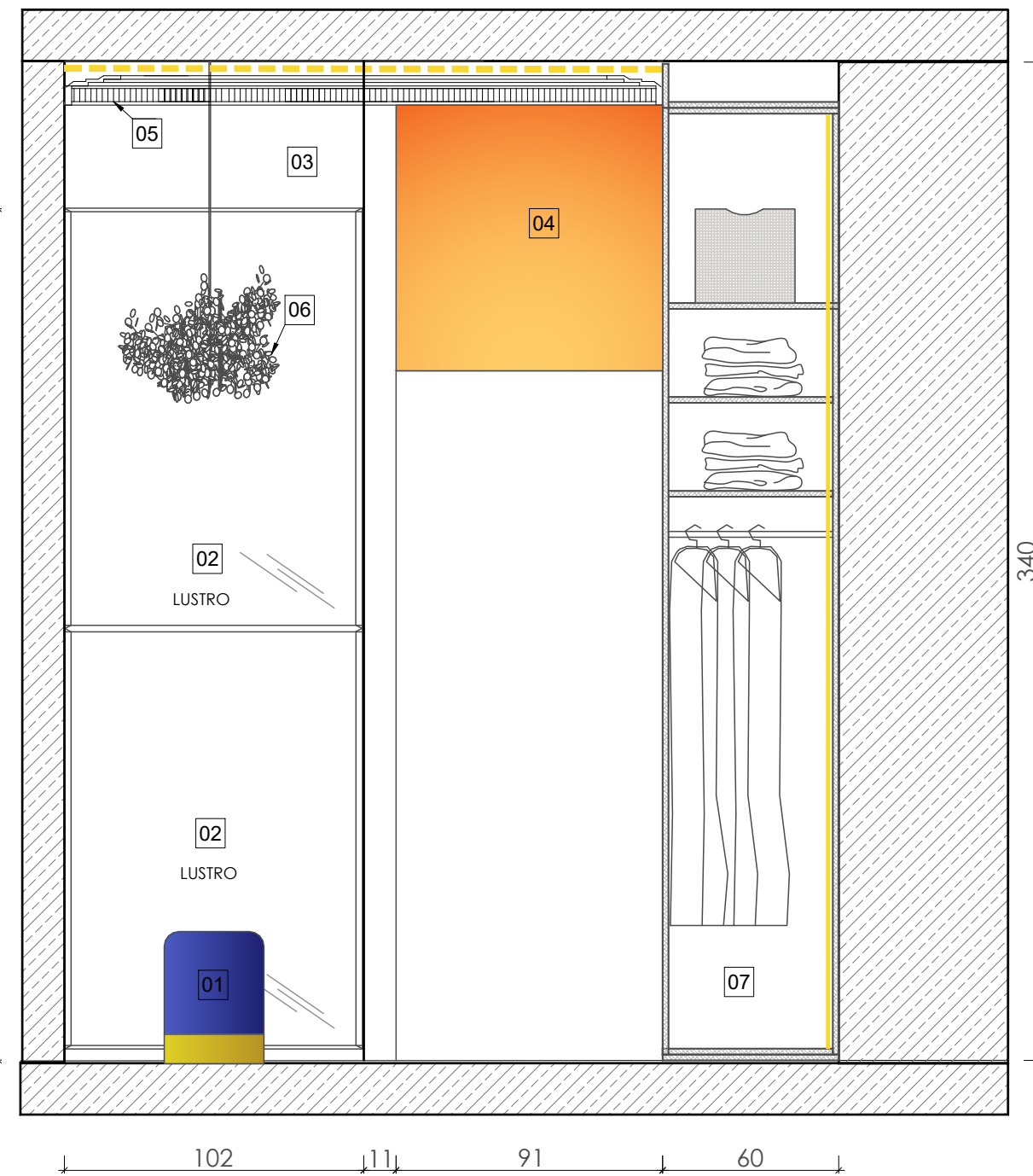
PRZEKRÓJ B-B
