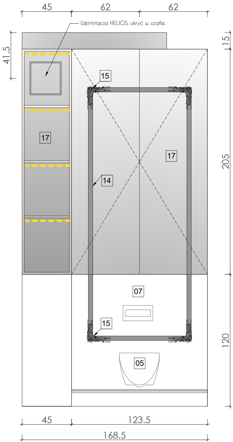
FRONT WIDOK
