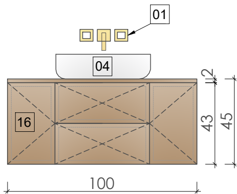
FRONT WIDOK
