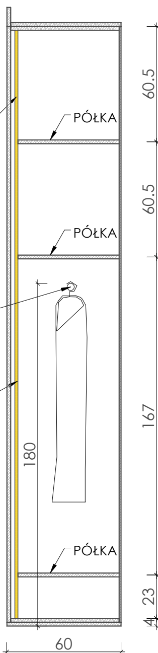
BOK SZAFY
