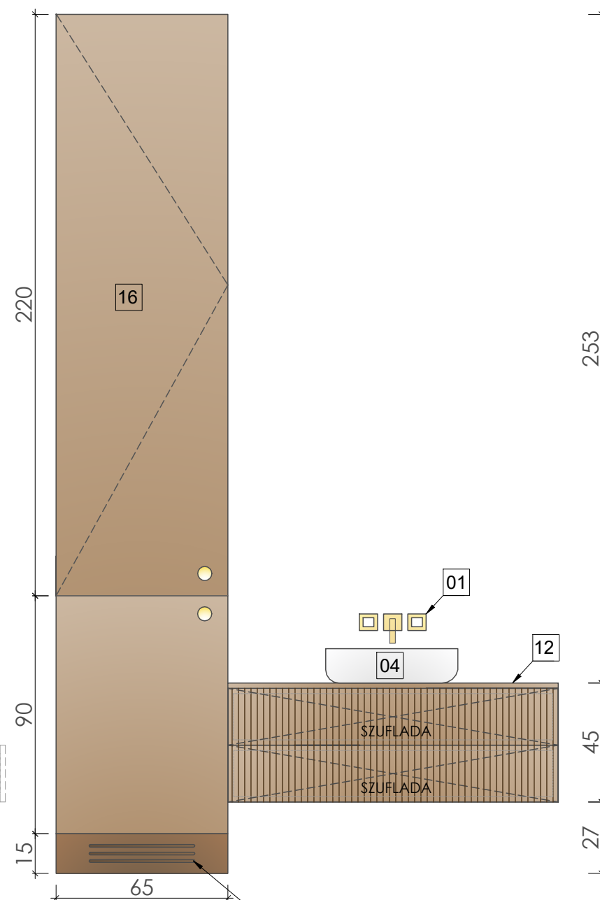
RZUT
