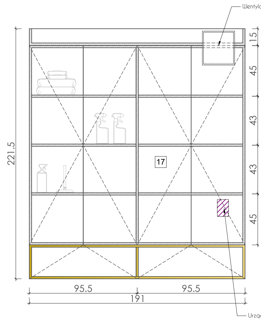
FRONT WNĘTRZE
