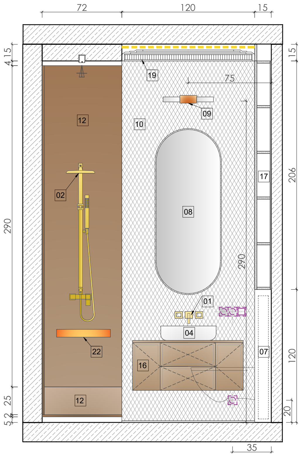
PRZĘKROJ B-B
