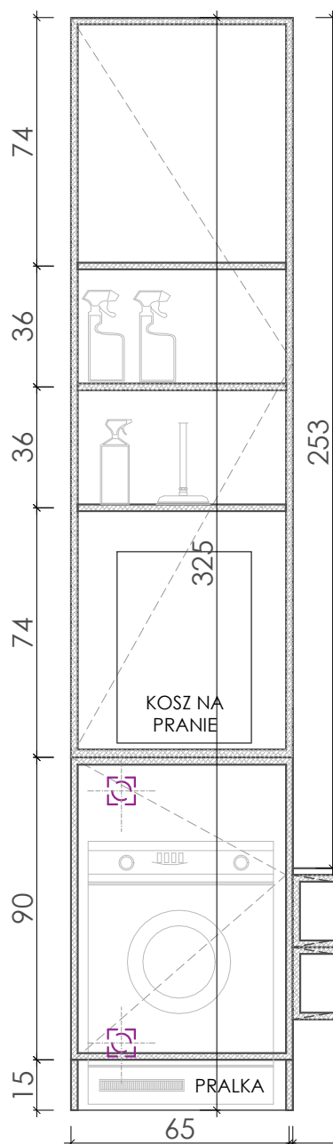
ZABUDOWA MEBLOWA NR 08
