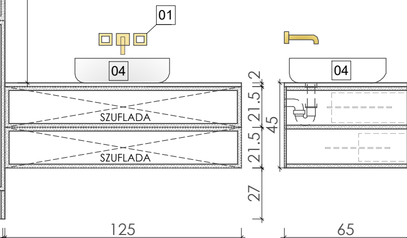
SZAFKA BOK WNĘTRZE
