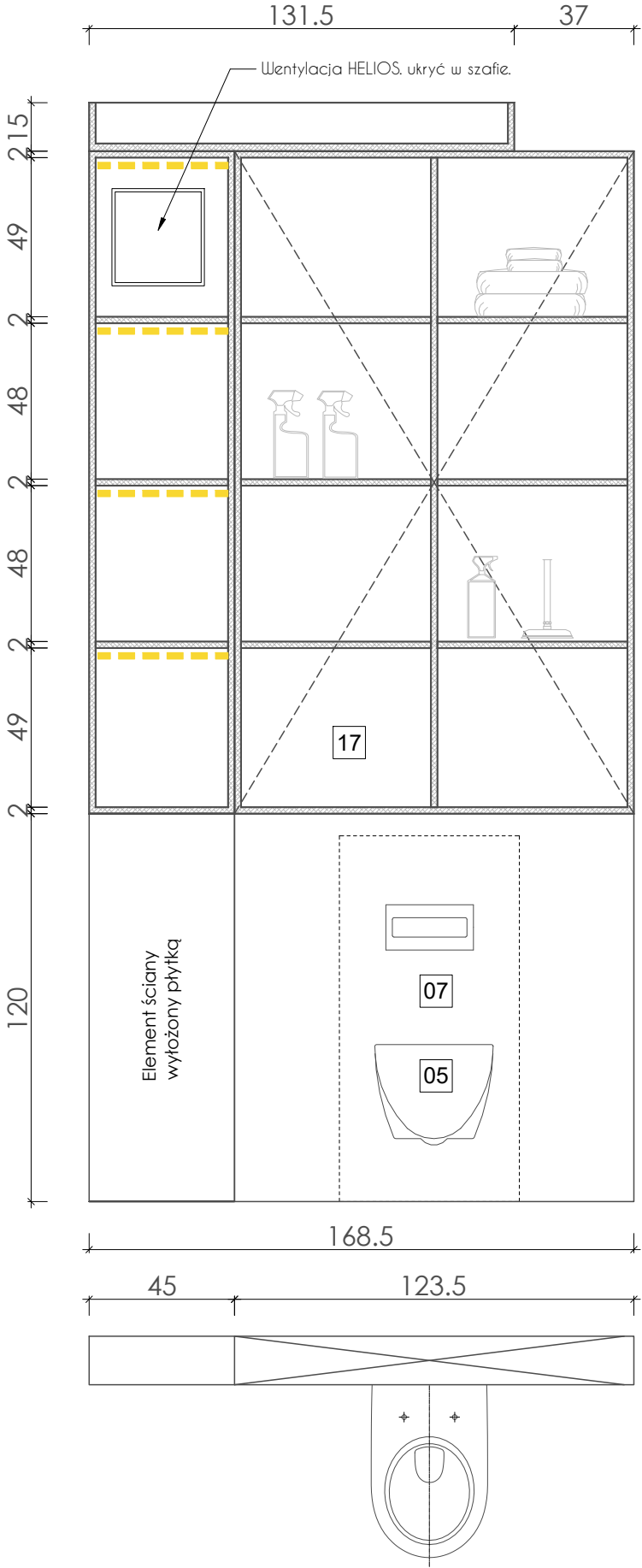
FRONT WNĘTRZE
