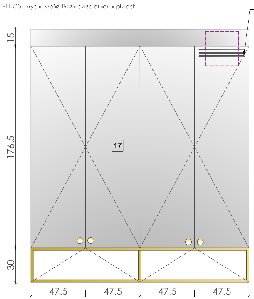
FRONT WIDOK
